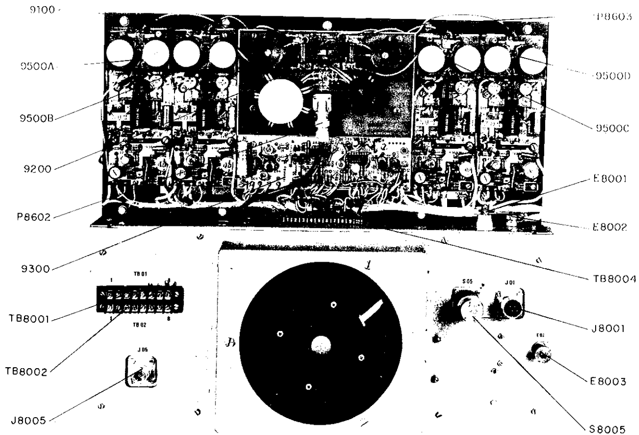
Fig. 2 - Vue arrière, capot supérieur déposé
